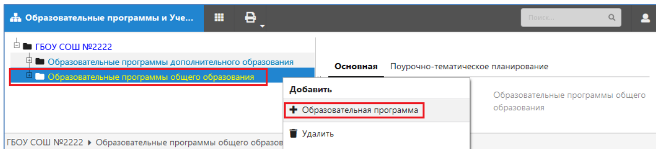
Рисунок 9. Добавление ОП
