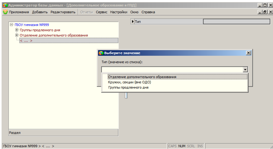
Рис. 3 Типы разделов
